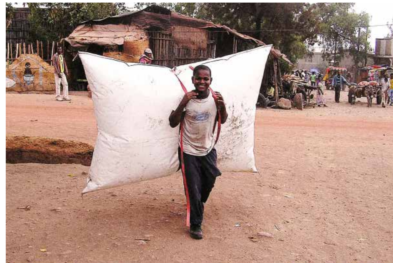
↑ Un esempio di "biogas backpack".
